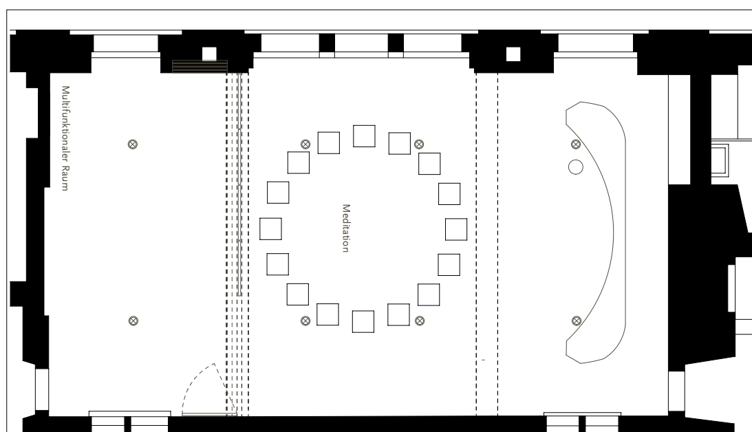
Grundriss des neuen Meditationsraumes und des kleineren multifunktionalen Raumes.
