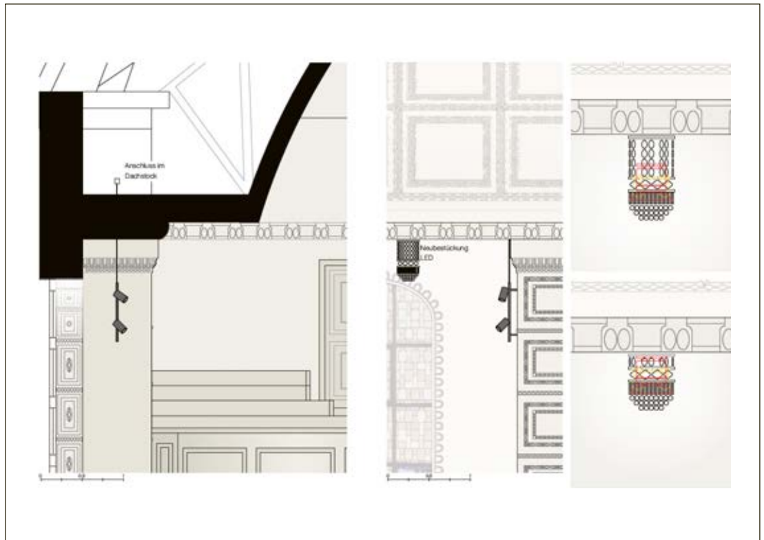
Details zur Neubestückung mit LED und Anbringung neuer Hochleistungsstrahler
